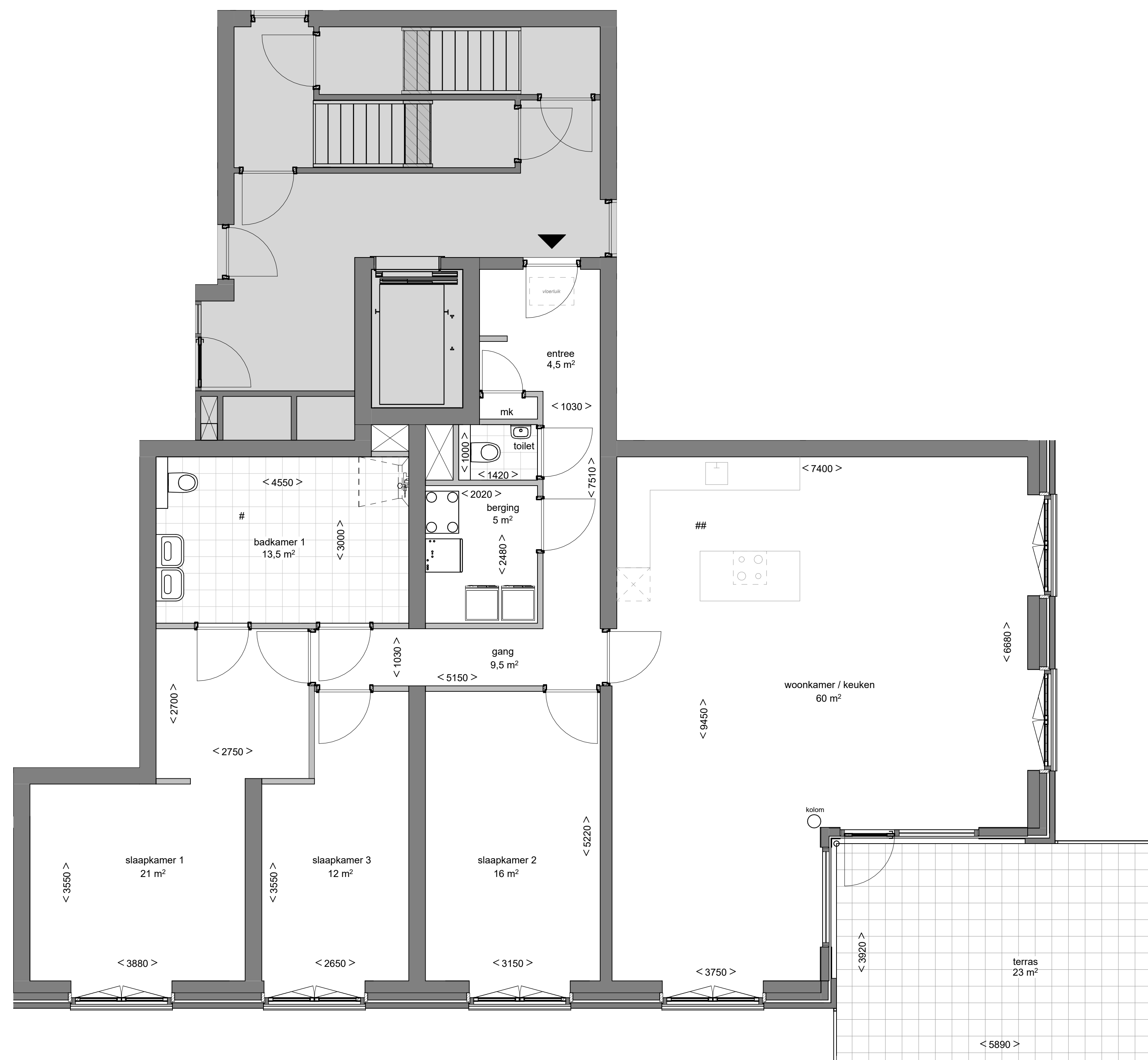
BEGANE GROND 1 : 50
