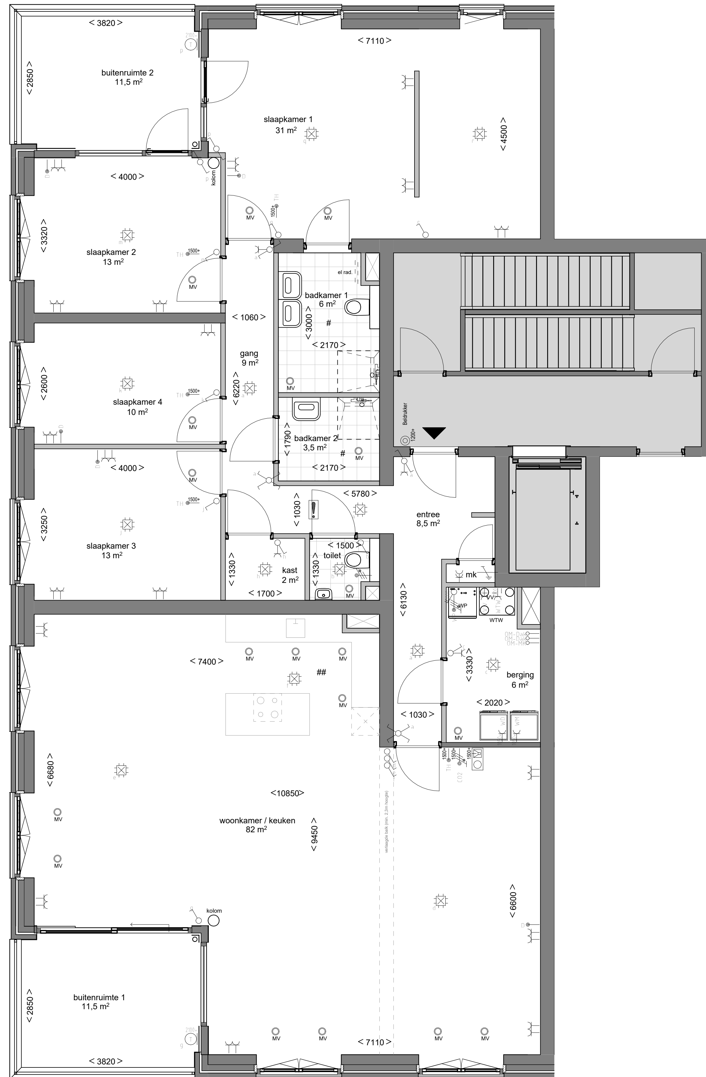
DERDE VERDIEPING 1 : 50
